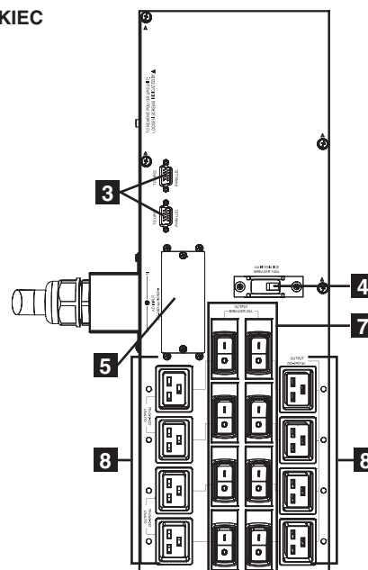
Panel posterior (válido para los 3 modelos)
